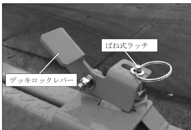
図9.4 - 作業床延長デッキロック
