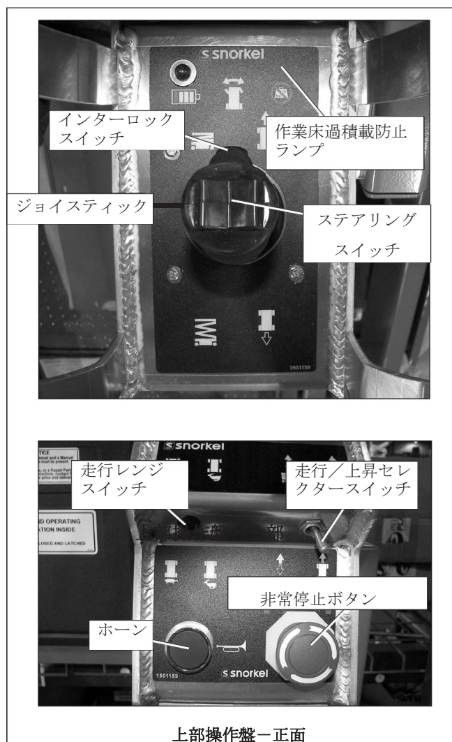
図9.2 - 上部操作盤
