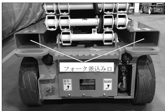
図10.1 - シャーシ後ろ側
