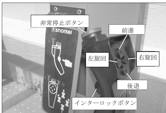
図9.3 - 積み込み操作盤
