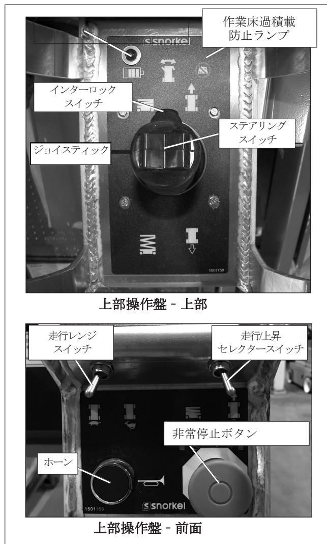
図7.3 - 上部操作盤
