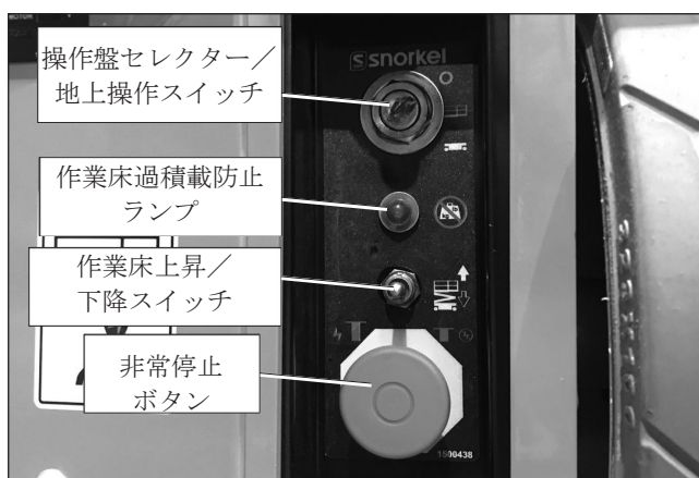
図9.1 - 下部操作盤
