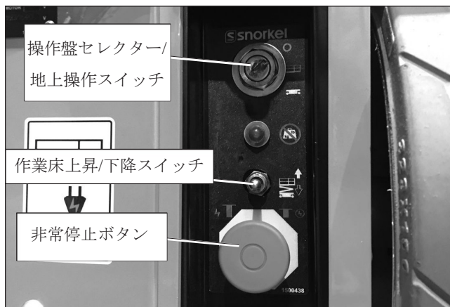
図8.8 - 下部操作盤
