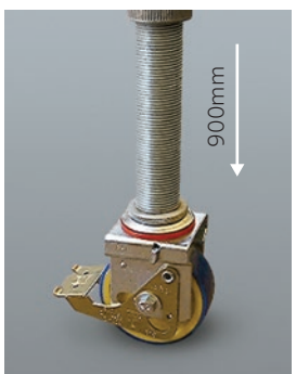
レッグは最大900mmまで伸び、段差に対応ができます。本体搬送時のキャスターは軸に対して偏心しておりハンドリングが軽快です。ロックすると直軸となり垂直荷重をしっかりと受けとめます。(プレーキ性能170kg)
