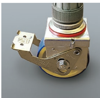
レッグは最大900mmまで伸び、段差に対応ができます。本体搬送時のキャスターは軸に対して偏心しておりハンドリングが軽快です。ロックすると直軸となり垂直荷重をしっかりと受けとめます。(プレーキ性能170kg)
